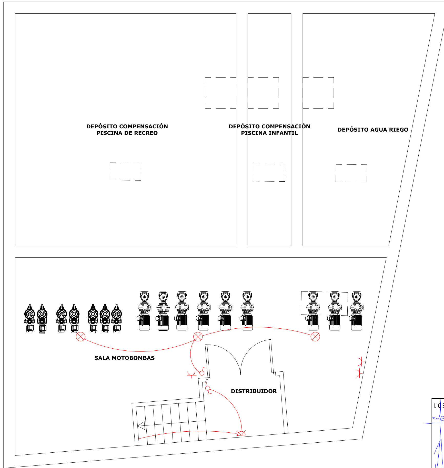
PLANTA SÓTANO
